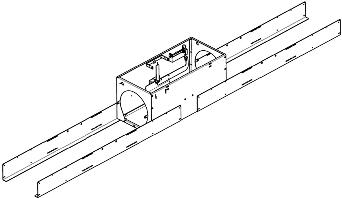
Abb. 5: Hauptkasten mit Grundrahmen
