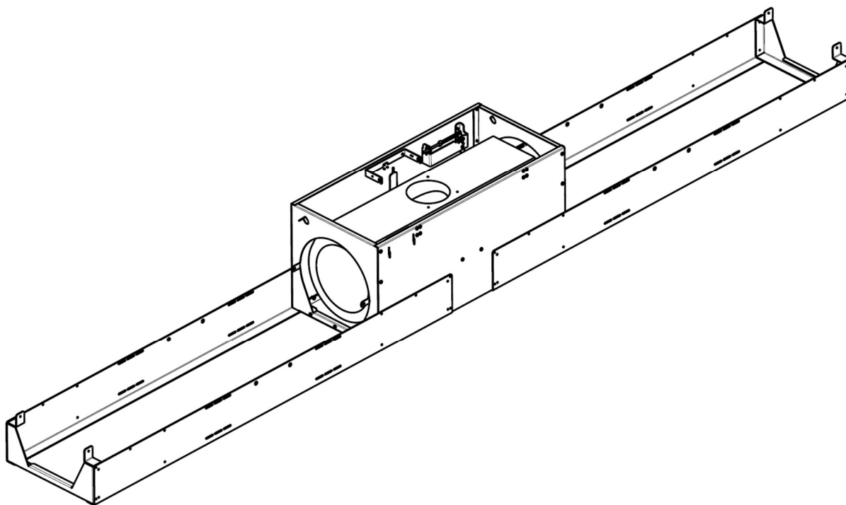
Abb. 11: In Waage ausgerichtetes Mittelrohr im Hauptkasten
