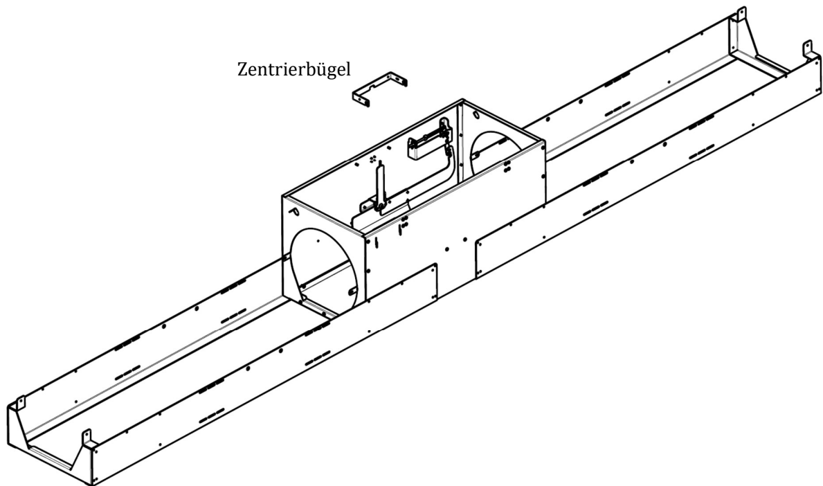
Abb. 6: Hauptkasten mit Grundrahmen und demontiertem Zentrierbügel
