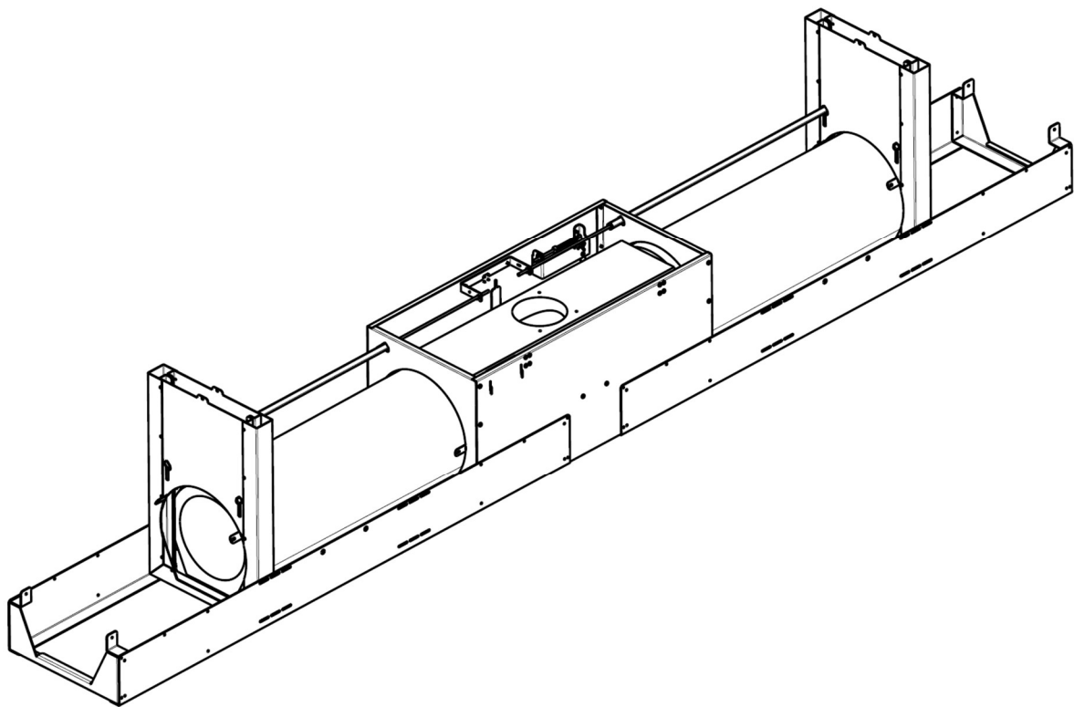
Abb. 14: Falle mit montiertem Gestänge
