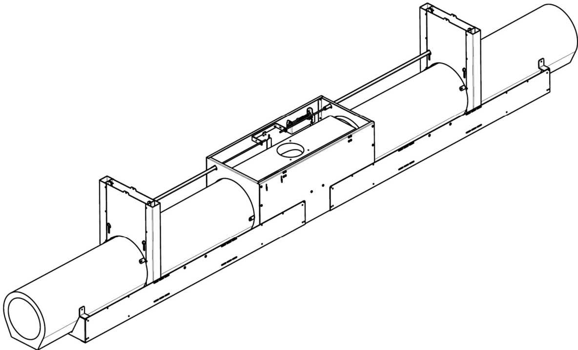
Abb. 16: Falle mit äußeren Anlegerohren
