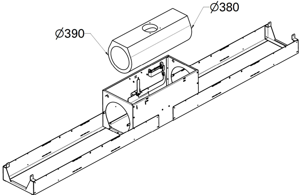
Abb. 10: Mittelrohrausrichtung zum Hauptkasten
