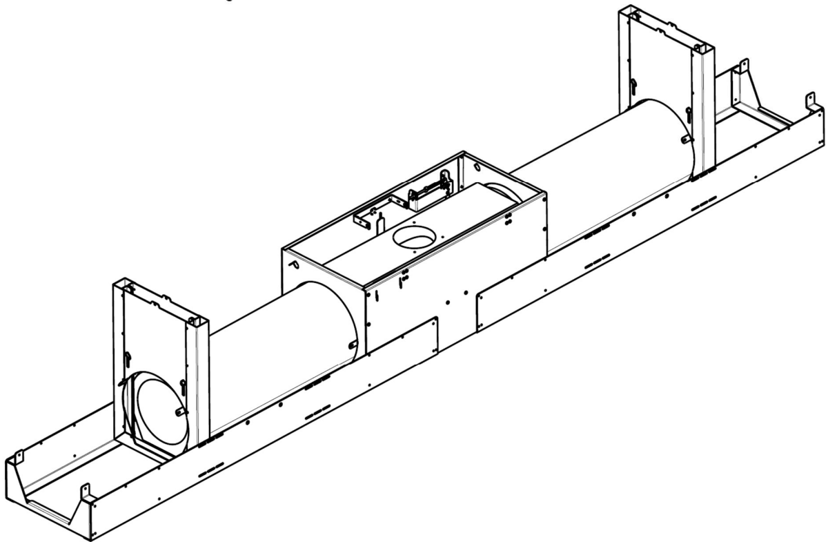
Abb. 13: Falle mit montierten Schieberkästen
